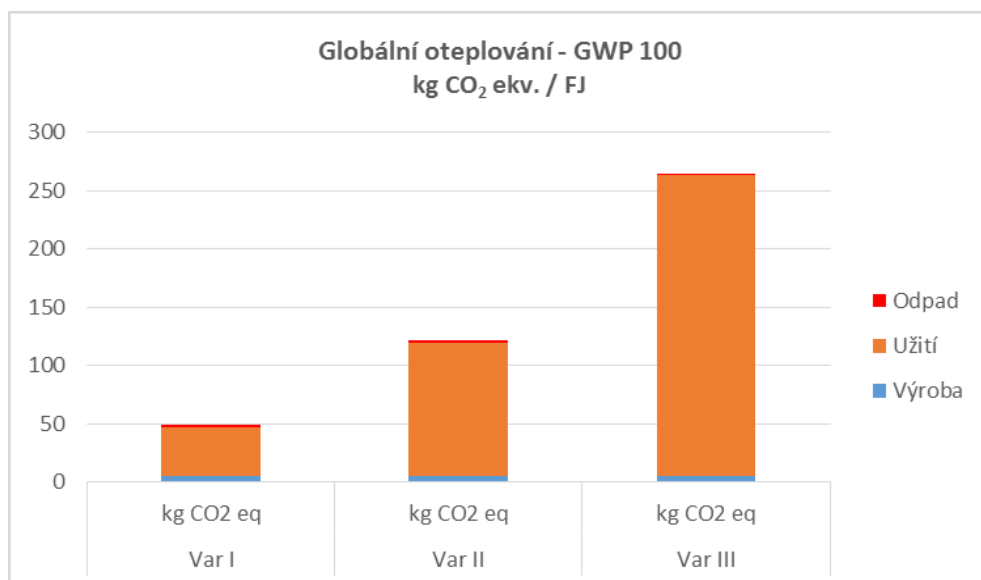
GRAF A3 KATEGORIE DOPADU GLOBÁLNÍ OTEPLOVÁNÍ – GWP 100 FOTOKATALYTICKÉHO NÁTĚRU FN2 VAR. I, II A III
