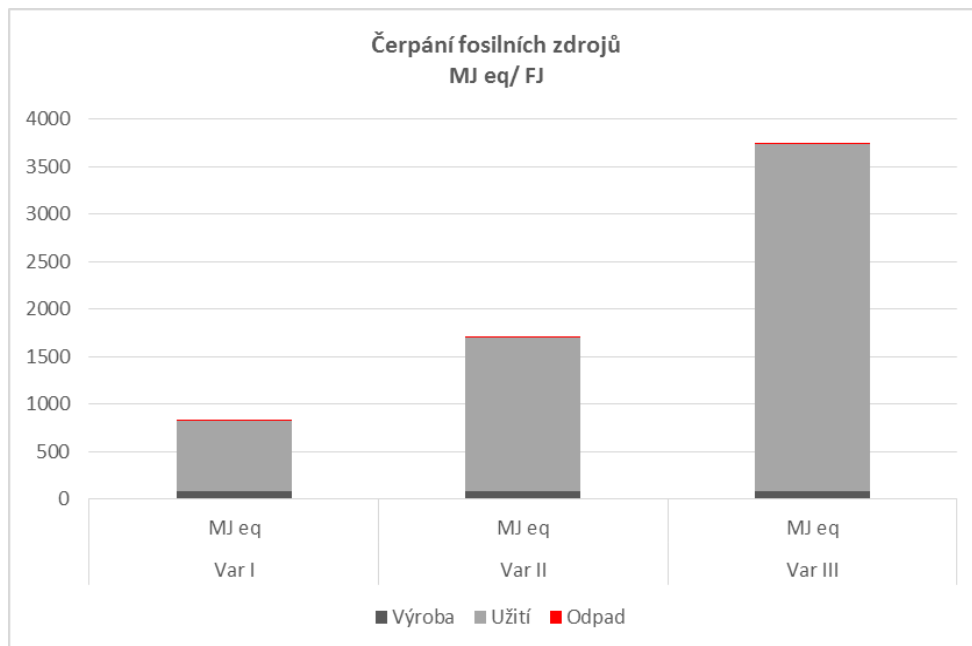
GRAF A4 KATEGORIE DOPADU ČERPÁNÍ FOSILNÍCH ZDROJŮ FOTOKATALYTICKÉHO NÁTĚRU FN2 VAR. I, II A III
