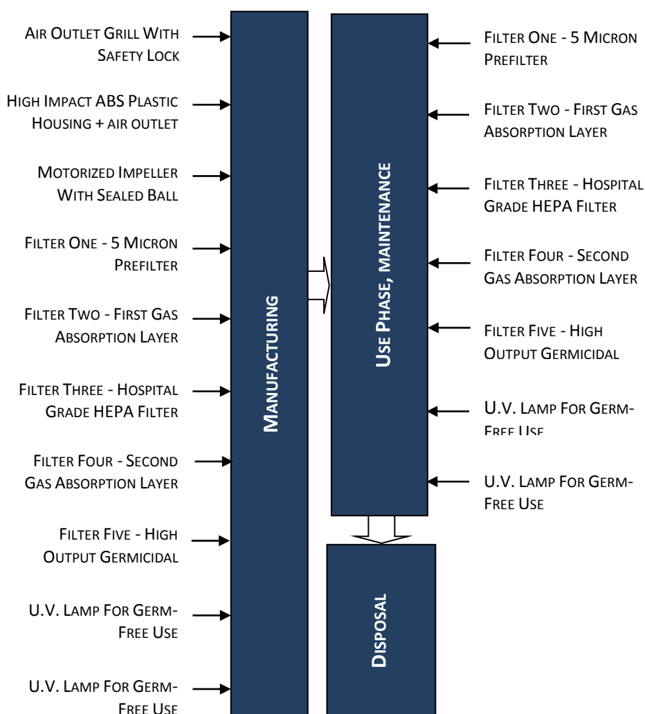
OBRAZEK 6 SCHÉMA ŽIVOTNÍHO CYKLU ČISTIČKY VZDUCHU - HRANICE SYSTÉMU
