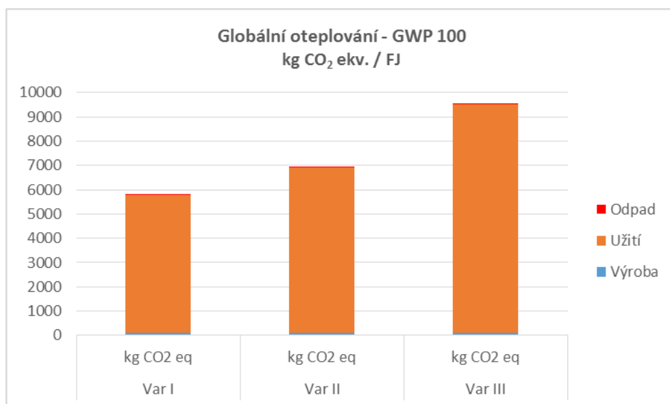
GRAF B3 KATEGORIE DOPADU GLOBÁLNÍ OTEPLOVÁNÍ – GWP 100 ČISTIČKY VZDUCHU VAR. I, II A III
