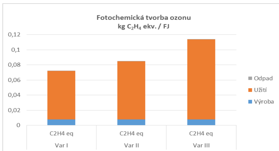
GRAF B7 KATEGORIE DOPADU FOTOCHEMICKÁ TVORBA OZONU ČISTIČKY VZDUCHU VAR. I, II A III
