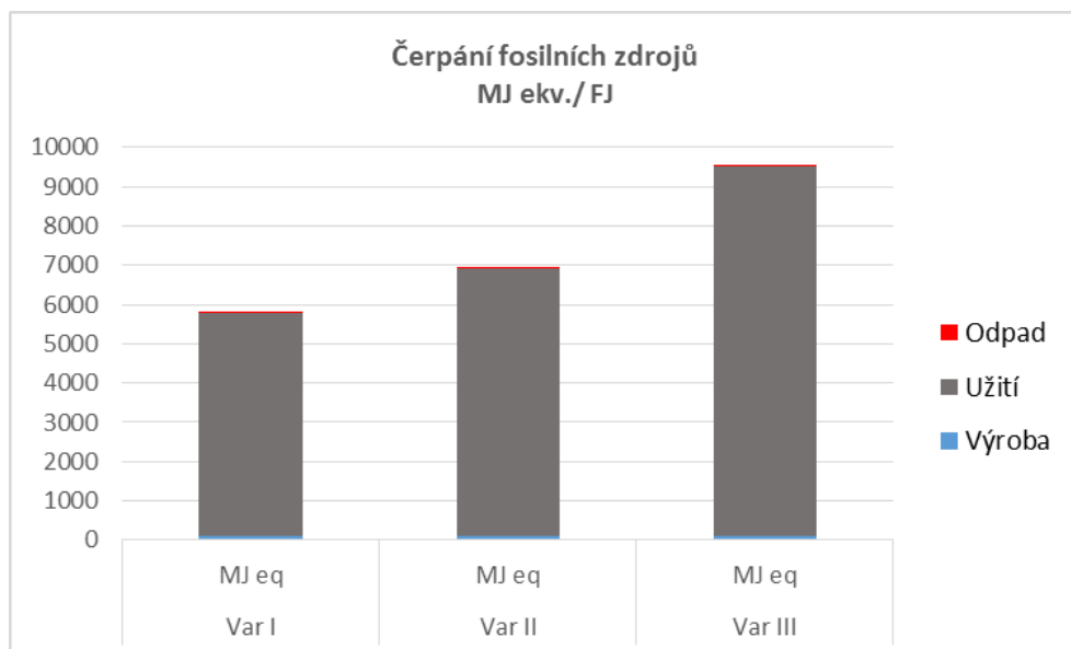
GRAF B4 KATEGORIE DOPADU ČERPÁNÍ FOSILNÍCH ZDROJŮ ČISTIČKY VZDUCHU VAR. I, II A III
