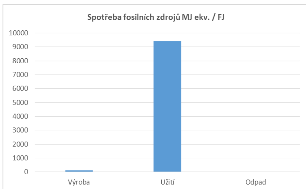
GRAF B2 KATEGORIE DOPADU SPOTŘEBA FOSILNÍCH ZDROJŮ ČISTIČKY VZDUCHU VAR. III
