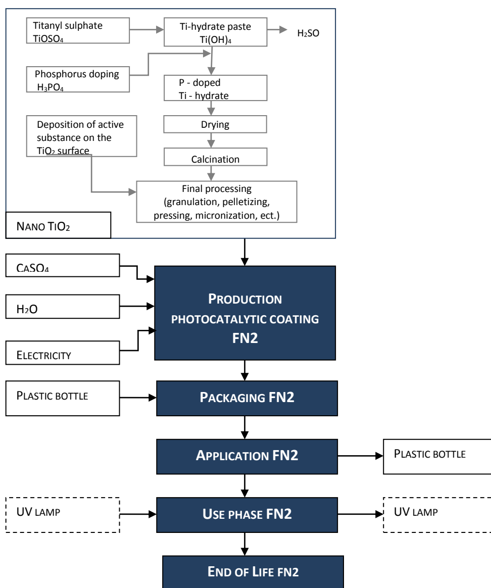
OBRAZEK 3 HRANICE ŽIVOTNÍHO CYKLU FN2
