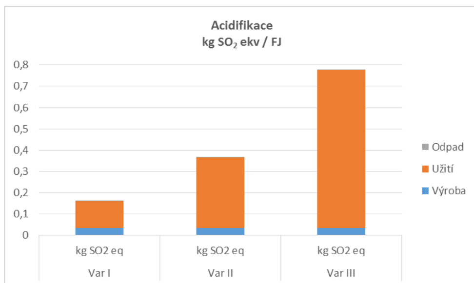
GRAF A6 KATEGORIE DOPADU ACIDIFIKACE FOTOKATALYTICKÉHO NÁTĚRU FN2 VAR. I, II A III
