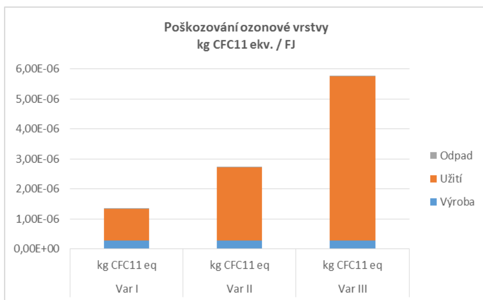
GRAF A5 KATEGORIE DOPADU POŠKOZOVÁNÍ OZONOVÉ VRSTVY FOTOKATALYTICKÉHO NÁTĚRU FN2 VAR. I, II A III
