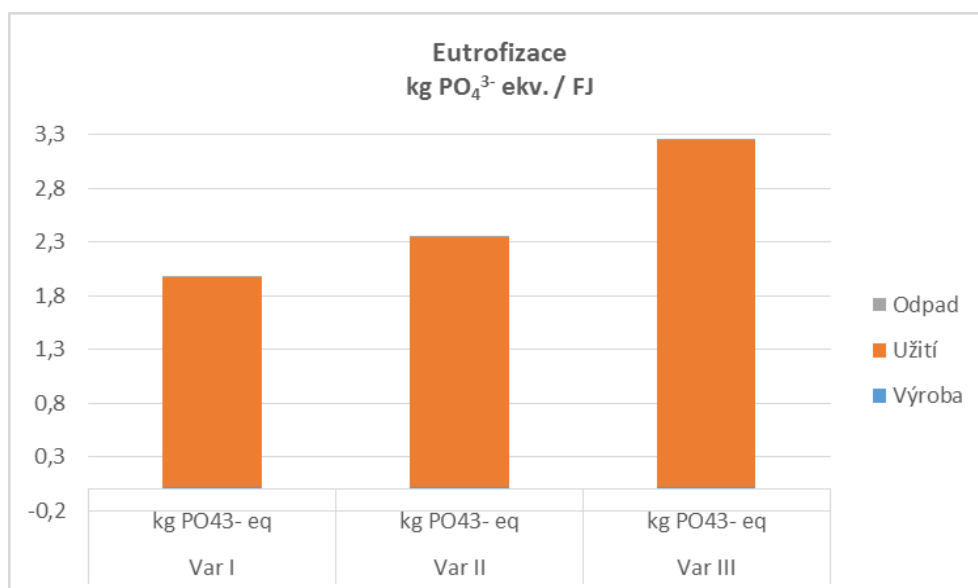
GRAF B8 KATEGORIE DOPADU EUTROFIZACE ČISTIČKY VZDUCHU VAR. I, II A III
