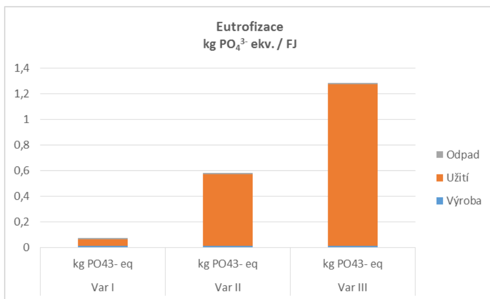
GRAF A8 KATEGORIE DOPADU EUTROFIZACE FOTOKATALYTICKÉHO NÁTĚRU FN2 VAR. I, II A III
