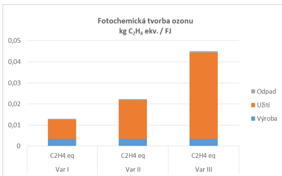
GRAF A7 KATEGORIE DOPADU FOTOCHEMICKÁ TVORBA OZONU FOTOKATALYTICKÉHO NÁTĚRU FN2 VAR. I, II A III
