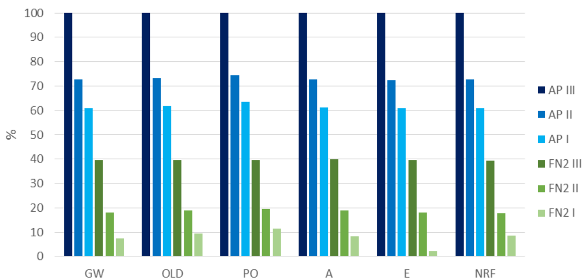
GRAF C1 POROVNÁNÍ VÝSLEDKŮ KATEGORIÍ DOPADU ČISTIČKY VZDUCHU A FOTOKATALYTICKÉHO NÁTĚRU FN2
